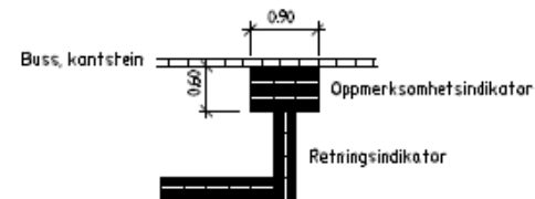
Detalj v / bussløyne og gangfelt
