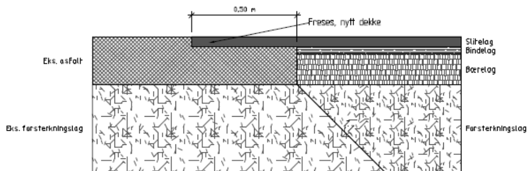
Prinsipp for tilkøbling mot eks. veioverbygning - I tverretning, snitt
