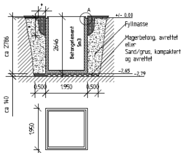
Figur - innbyggingsplan
