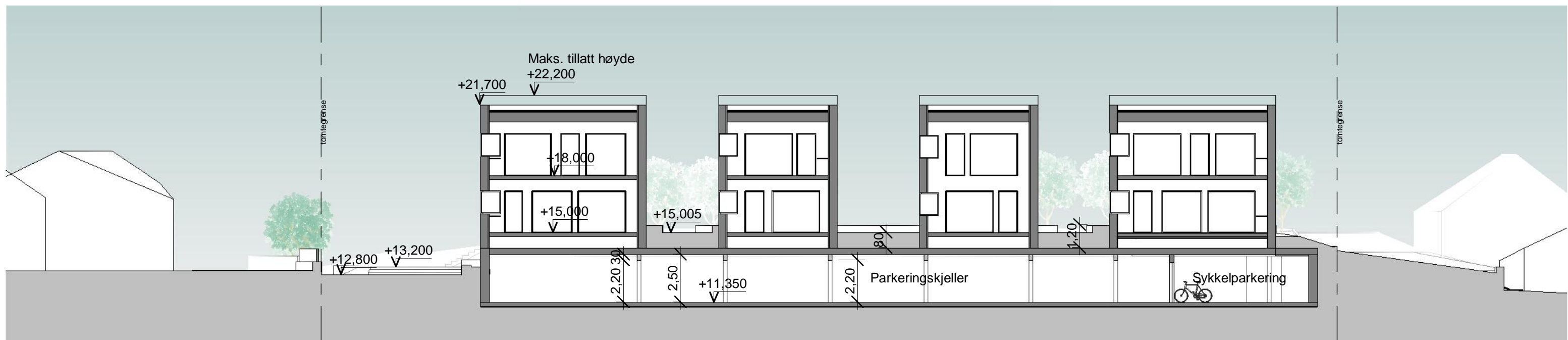
Snitt B 1 : 200
