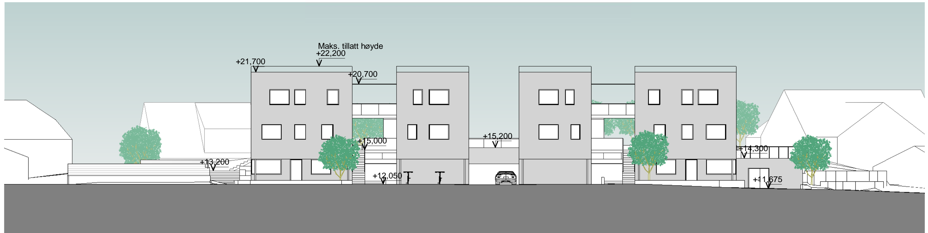
Sør-Øst 1 : 200
