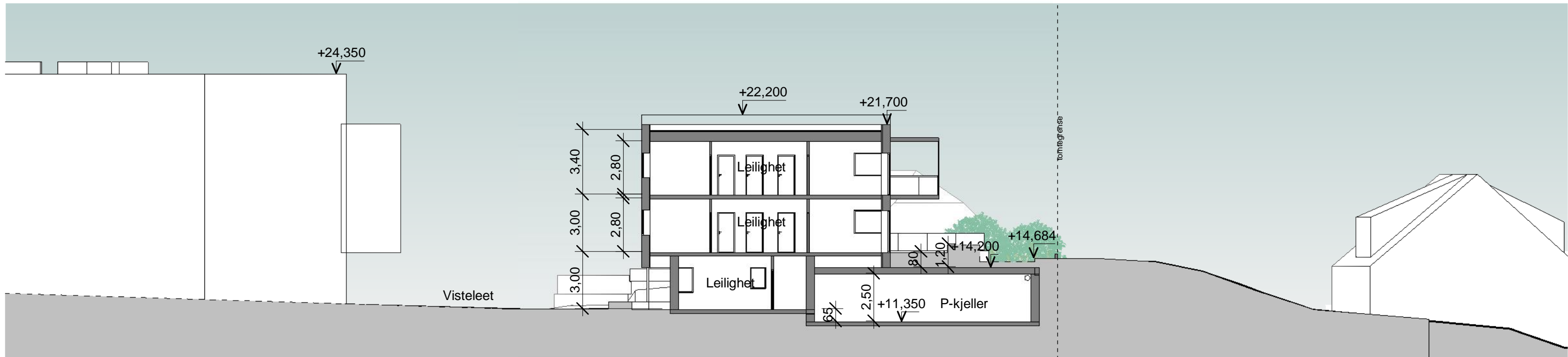
Snitt A 1 : 200
