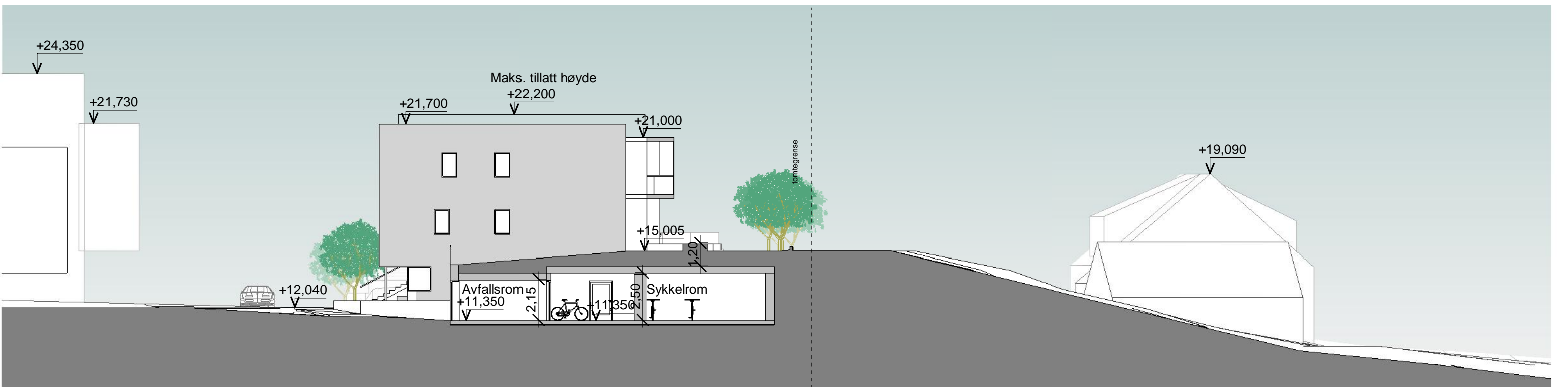
Nord-øst 1 : 200
