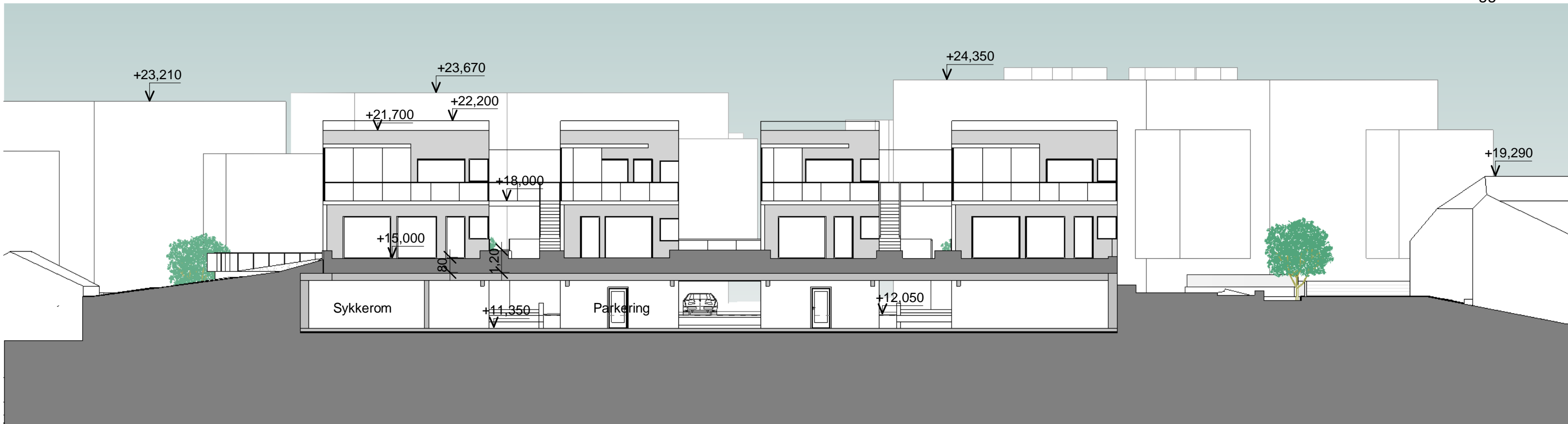
Nord-vest 1 : 200
