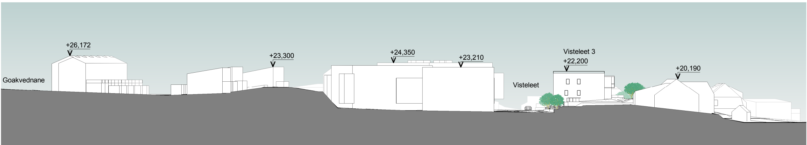
Overordnet snitt 1 : 500
