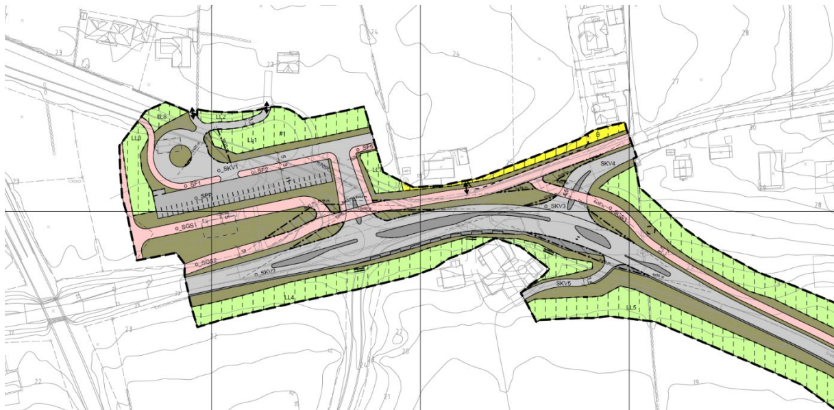
Figur 12 Omlagt kryss
